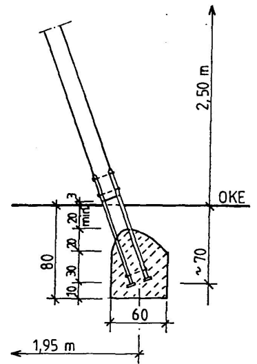
Schnitt Ausführung m. Pfostenschuhen
